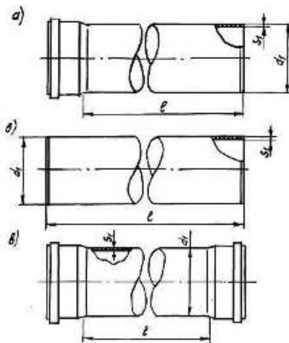
Рисунок 1. Трубы.
